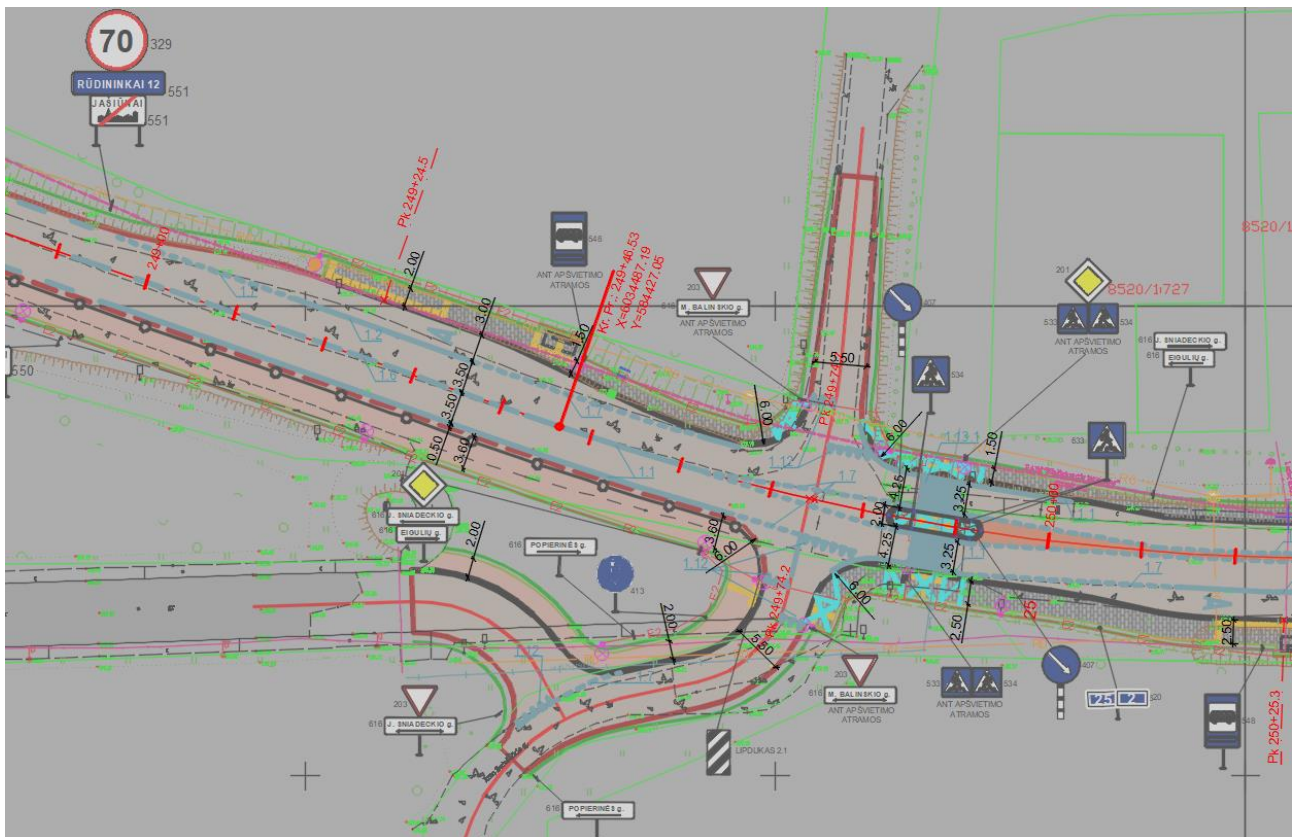
4 pav. 24,967 km sankryžos schema
