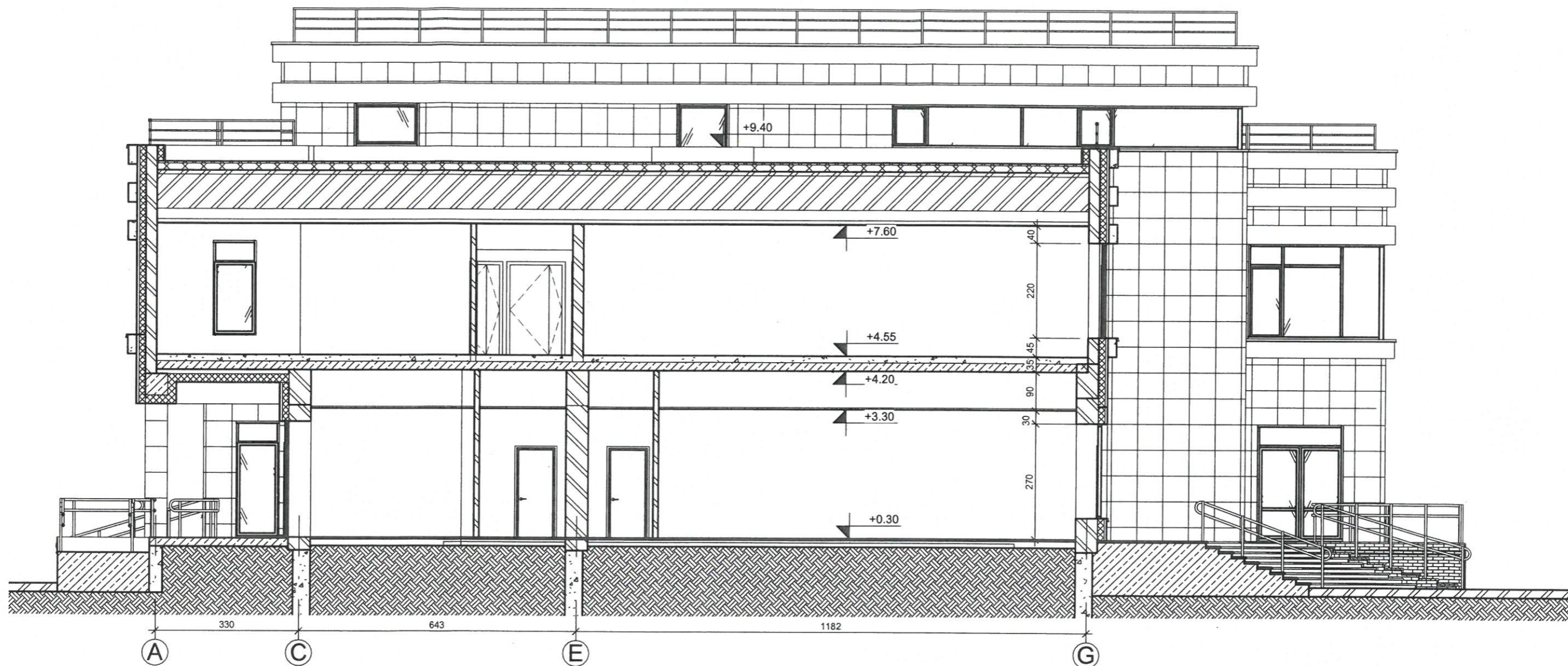
Pjuvis A-A M1:100
